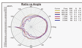
PH-150指向性(极坐标)
