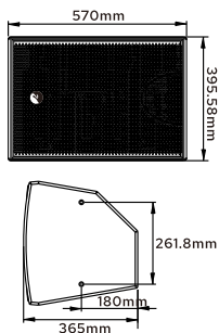
PH-350尺寸图
