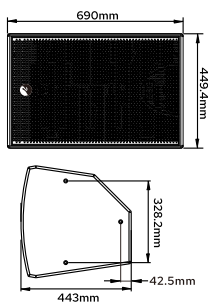
PH-550尺寸图
