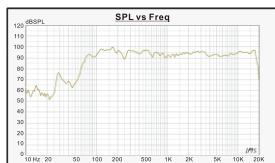
PH-150频响曲线
