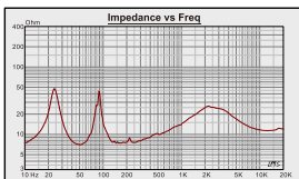
PH-550阻抗曲线
