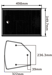
PH-150尺寸图
