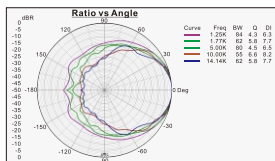
PH-550指向性(极坐标)
