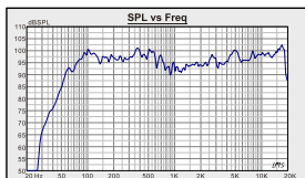
PH-550频响曲线
