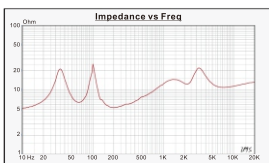
PH-150阻抗曲线
